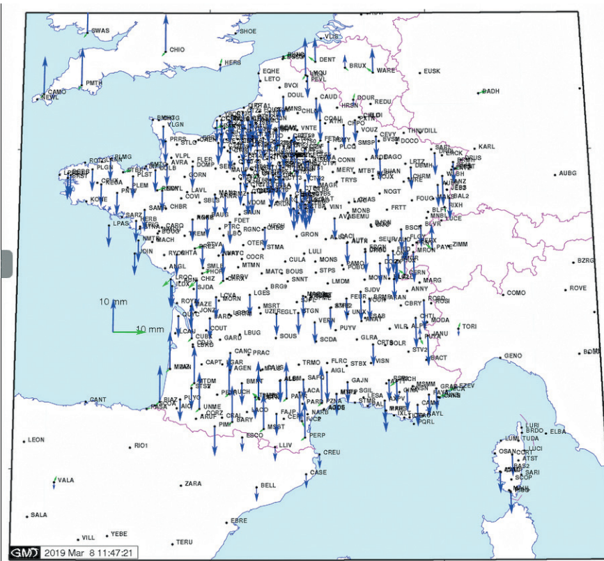
Figure 1. Changements de coordonnées théoriques dus aux changements de calibrations d'antenne lors de la parution de l'ITRF2014.
