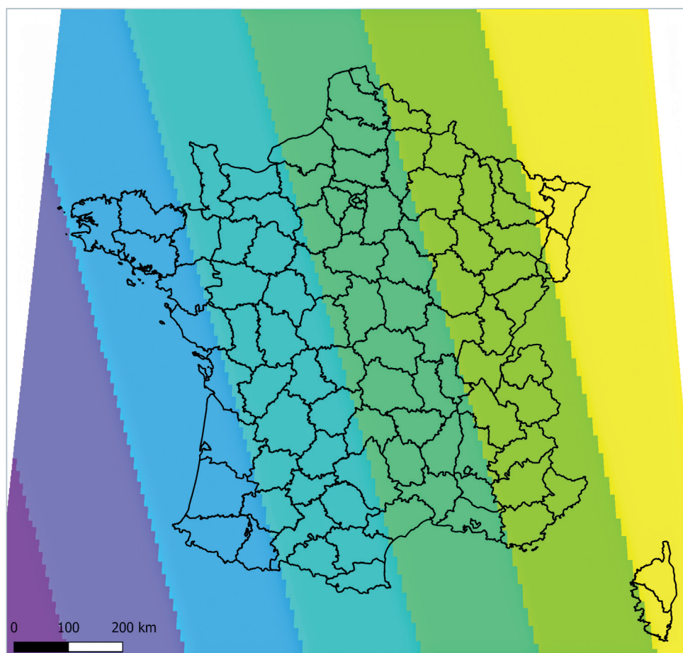
Figure 5. Écarts (en mm) entre RGF93v2b et RGF93v2 sur la composante verticale.
